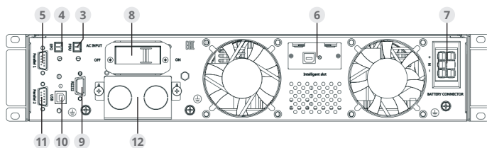
Вид сзади
