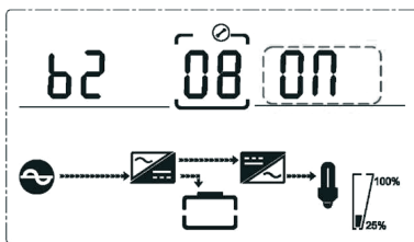
Настройка отключения звуковой сигнализации (Примечание: часть изображения, выделенная пунктиром, мигает).
