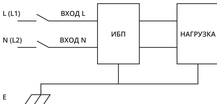
Входное соединение «одна фаза + земля»
