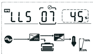
Настройка минимального напряжения байпаса (Примечание: часть изображения, выделенная пунктиром, мигает).
