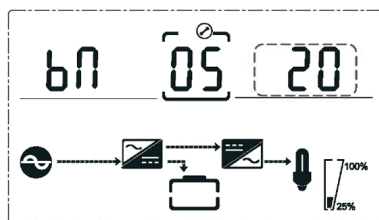
Настройка количества АКБ
