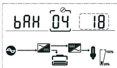
Настройка емкости АКБ
