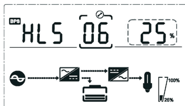
Настройка максимального напряжения байпаса (Примечание: часть изображения, выделенная пунктиром, мигает).
